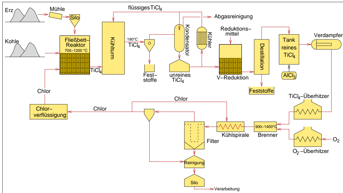
Anlagen-Schema Chlorid-Prozess
