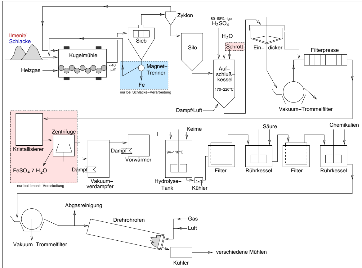
Anlagen-Schema Sulfat-Prozess
