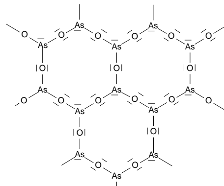
Struktur von Claudetit As 2 O 3
