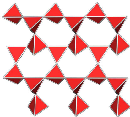
Struktur von O-P 2 O 5
