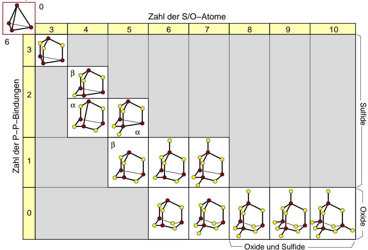
Struktursystematik von P-Oxiden und -Sulfiden
