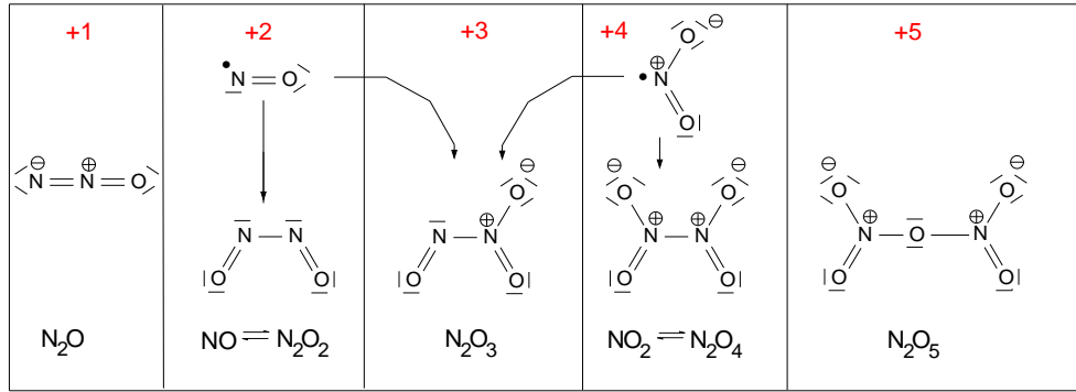
Valenzstrichformeln der Stickoxide (nach Oxidationsstufen am N)
