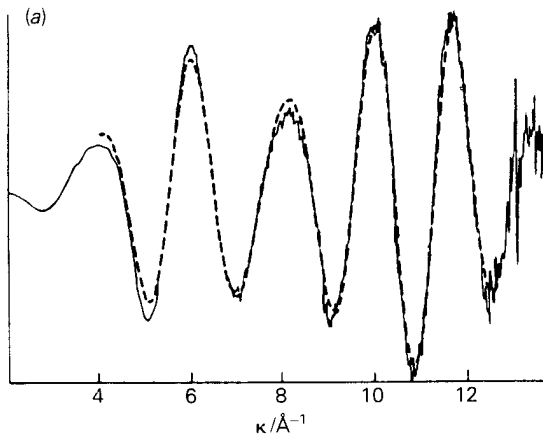
EXAFS-Daten κ 3 χ(κ)
