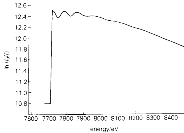
Röntgenabsorptionsspektrum (Co K-Kante) von Co 2 (Pφ 2 ) 2 cp 2
