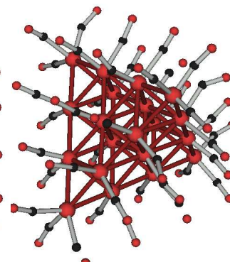
[Os_{20}(CO)_{40}]^{2-}
