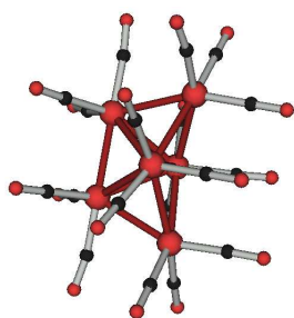
Os_6(CO)_{18}
