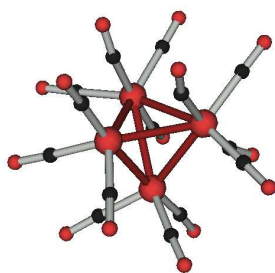
Os_4(CO)_{14}
