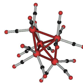
Os_5(CO)_{16}
