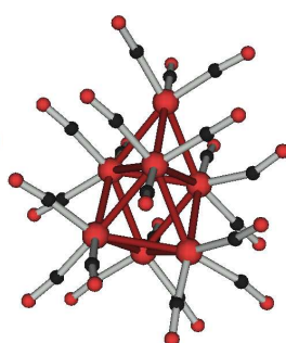
Os_7(CO)_{21}
