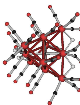
[Os_{10}C(CO)_{40}H_2]
