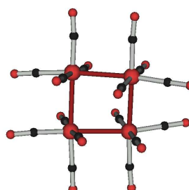
Os_4(CO)_{16}
