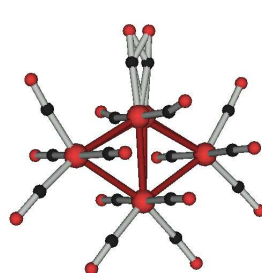
Os_4(CO)_{15}
