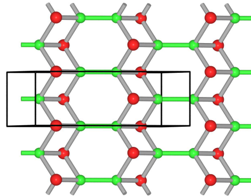
InSe
