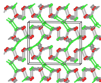
In 4 Se 3
