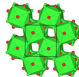
Tl 5 Se 3
