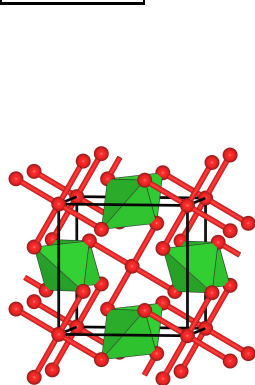
Ga 2 Te 5
