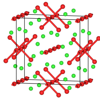
TlTe
