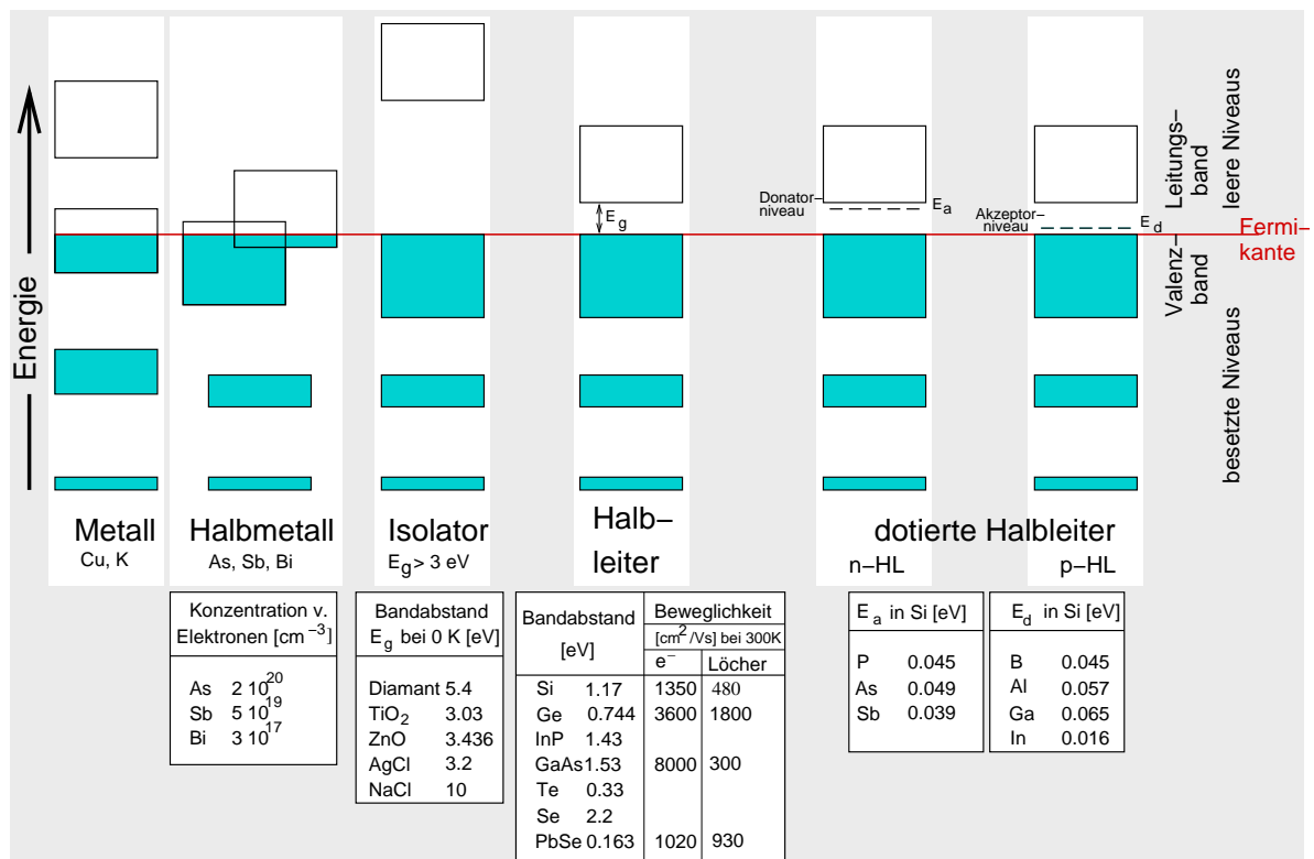
vereinfachte Zustandsdichten verschiedener Festkörper
